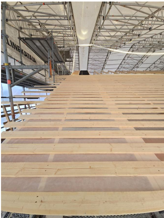
Vesikaton puutyöt käynnissä, kattoristikot asennettu. Aluskatteen ja ruodelautojen asennus käynnissä
