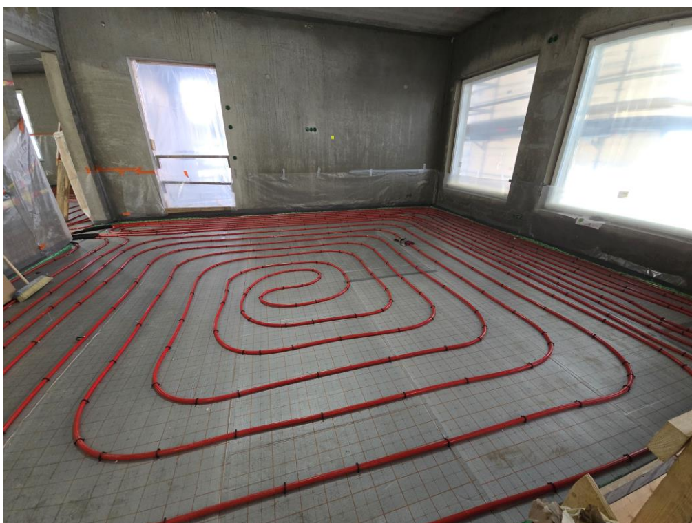
2. krs lattialämmityksiä asennettuna
