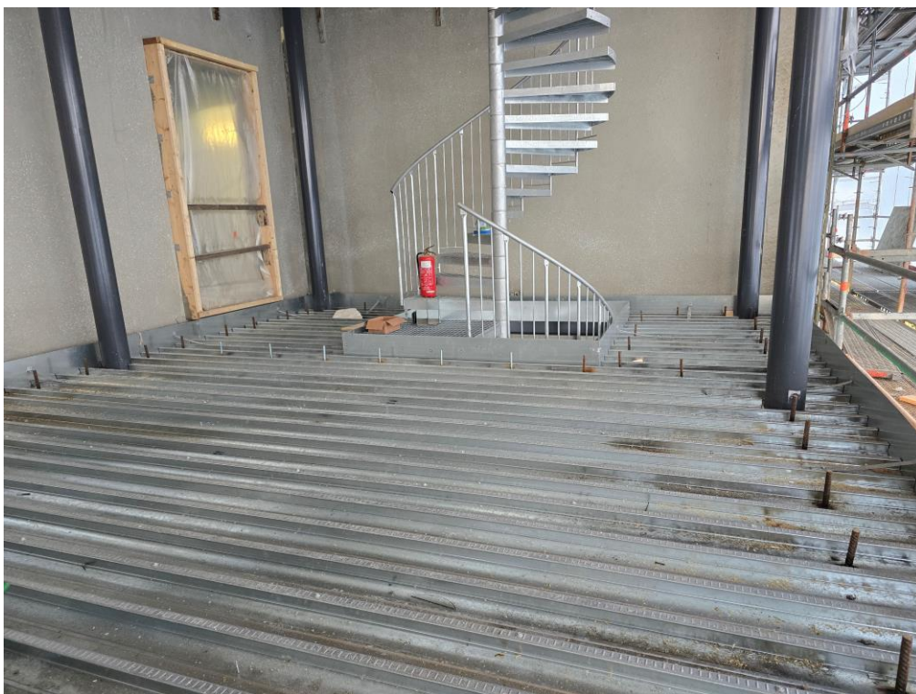
Parvekkeen teräsrakenteet asennettu ja kierreportaan asennus aloitettu
